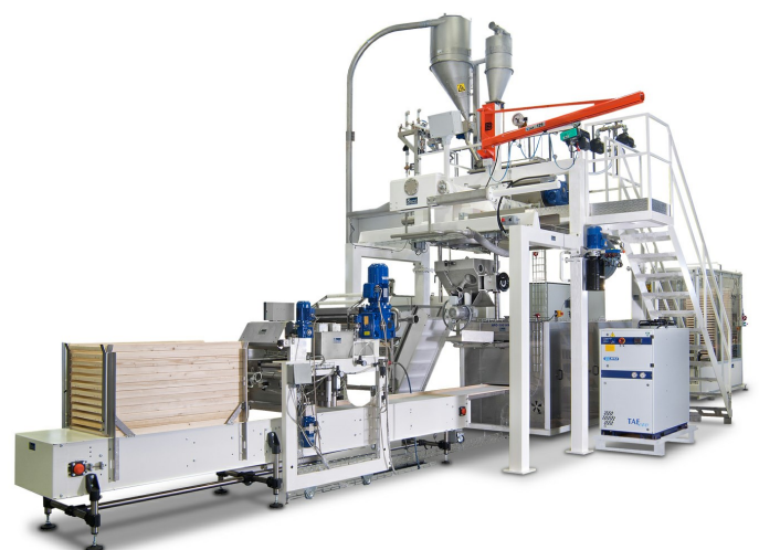
Linea speciale per nidi, lasagne, paste corte e speciali
